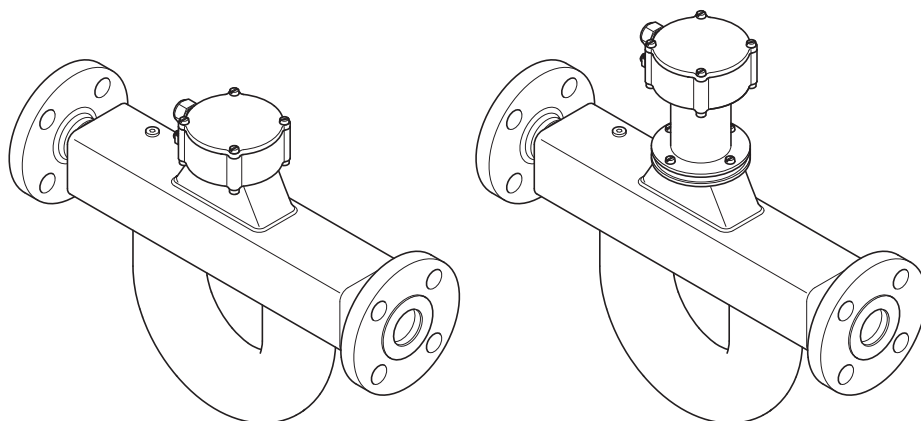
図 17: 分離形検出器，端子箱標準形および端子箱距離延長形，流量計サイズ 34，36 および 38
