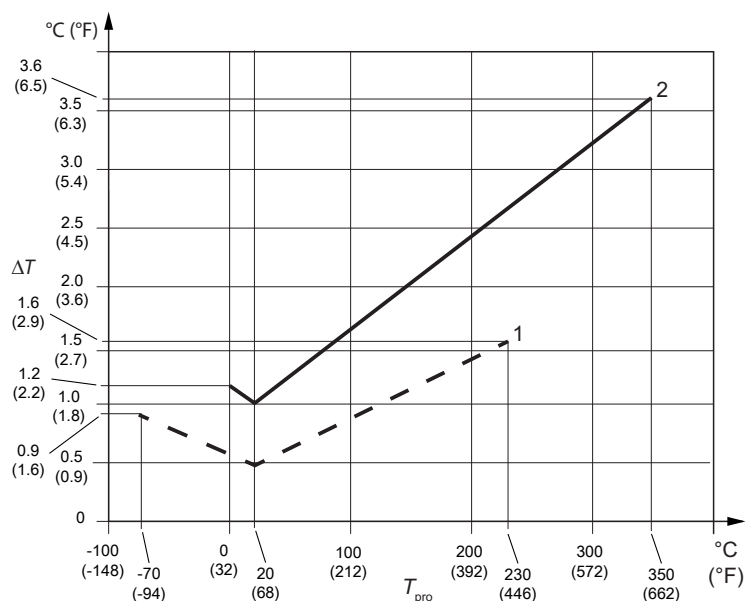
図 6: 温度の精度
