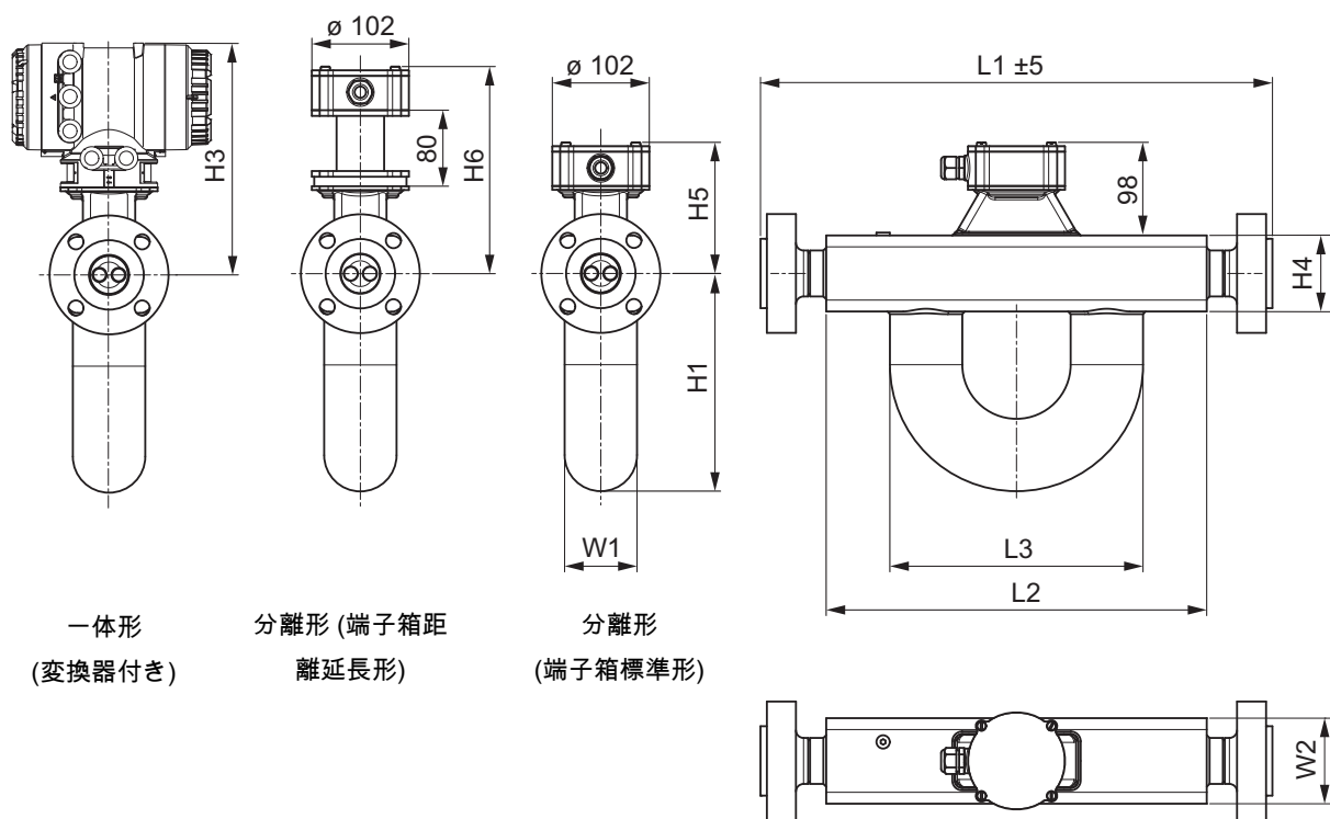
図 19: 寸法 (単位 mm)
