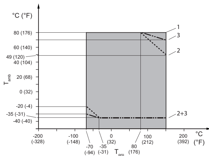
図 13: 許容される流体温度および周囲温度 (分離形)
