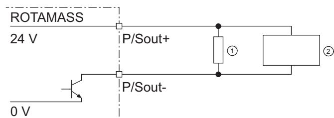
図 28: アクティブパルス出力接続 P/Sout の接続図
