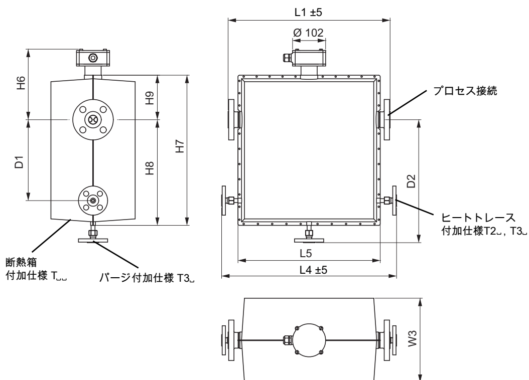
図 20: 流量計サイズ Intense 34, 36 および 38 の寸法 (単位 mm):断熱箱付き
