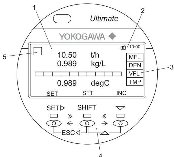
図 41: 表示器のレイアウト
