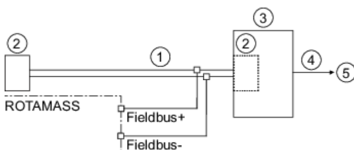
図 39: PROFIBUS PA 接続
