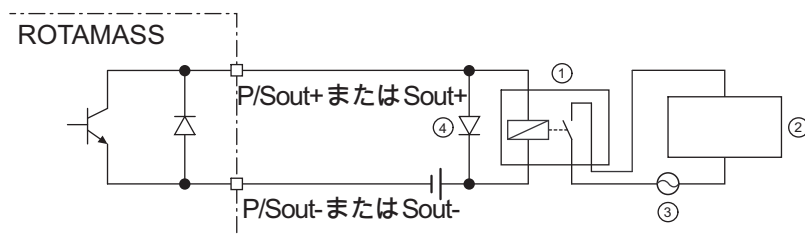
図 36: ソレノイドバルブ回路がある場合のパッシブステータス出力接続 P/Sout または Sout の接続図
