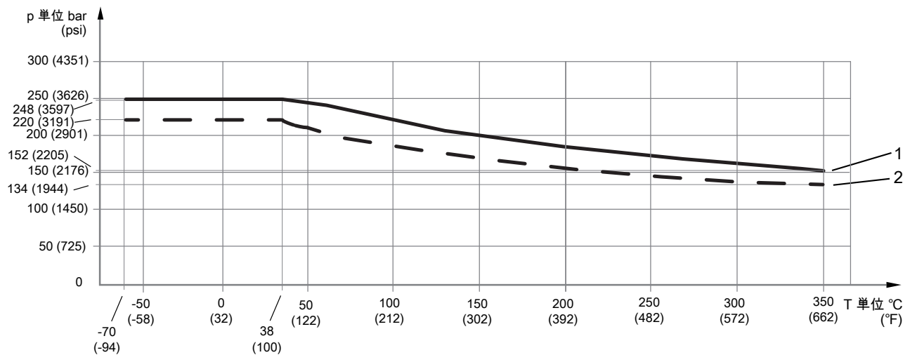
図 9: プロセス接続部の温度と許容プロセス圧力の関係
