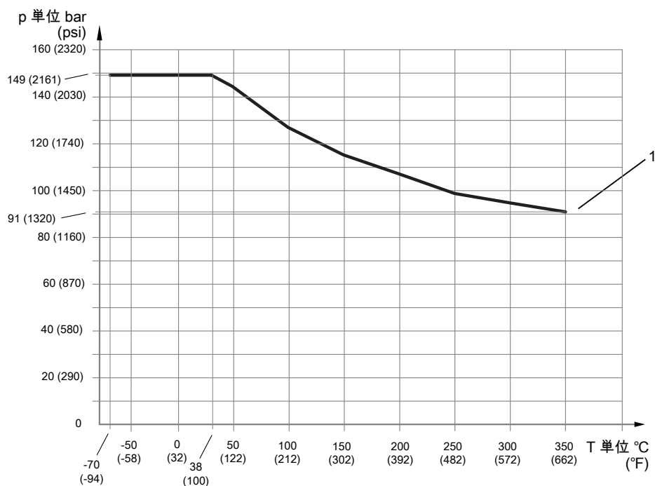
図 8: プロセス接続部の温度と許容プロセス圧力の関係
