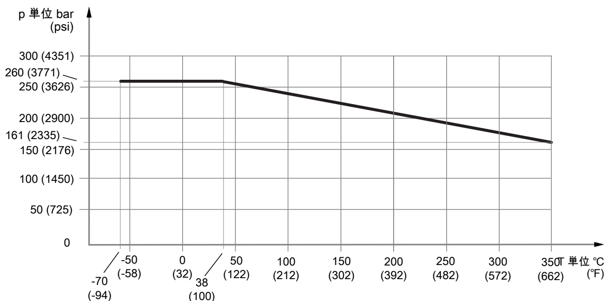
図 10: 温度の関数として表される許容プロセス圧力
