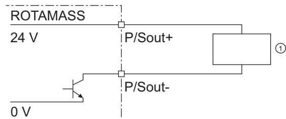
図 33: アクティブステータス出力接続 P/Sout
