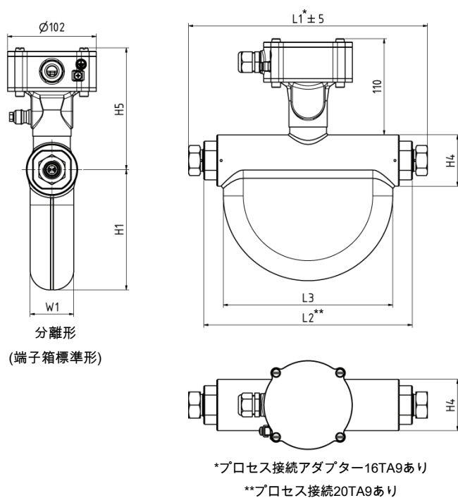
図 18: Intense 08 および 10 の寸法 (単位 mm)
