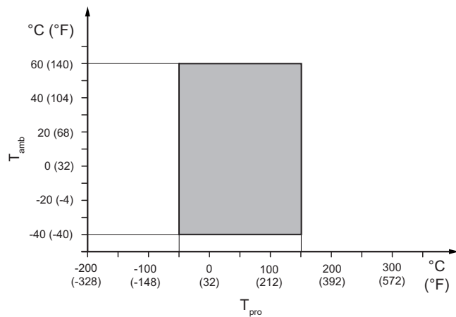
図 12: 許容されるプロセス流体温度および周囲温度 (一体形)
