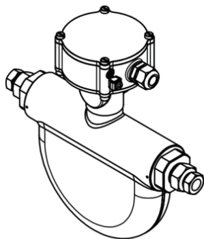
図 16: 分離形検出器，端子箱標準形，流量計サイズ 08 および 10
