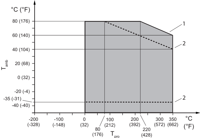
図 15: 許容される流体温度および周囲温度 (分離形)
